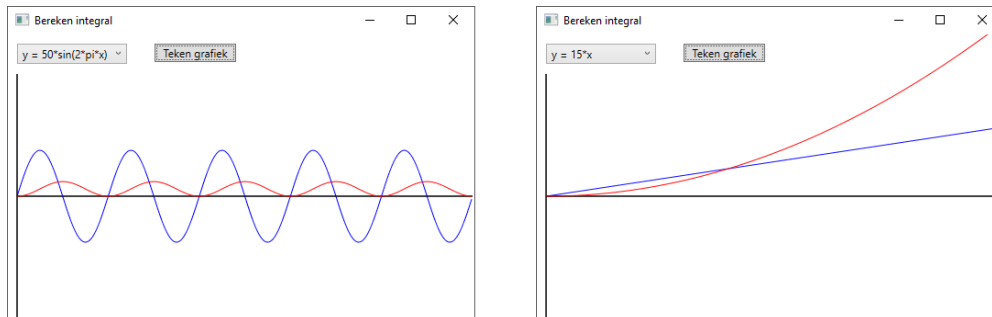
Figuur 2: Voorbeeld van het programma. De rode lijn stelt de integraal voor, terwijl de blauwe lijn de originele functie voorstelt.
